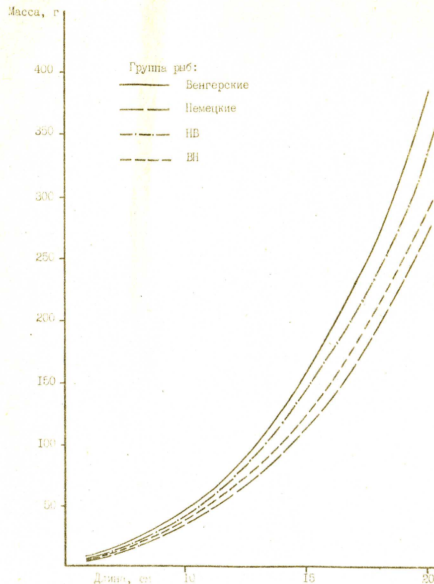
Рис. 2. Зависимость между длиной ( l ) и массой ( P ) тела у карпов различного происхождения
