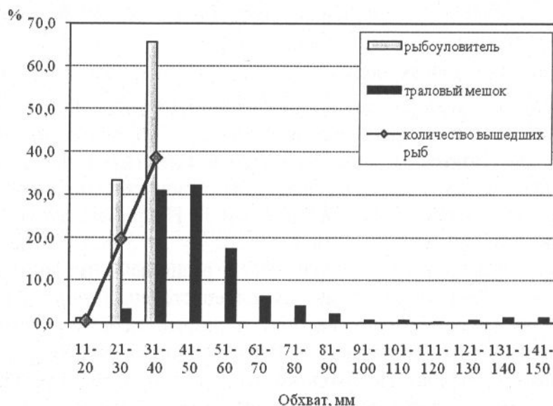
Рис. 2. Распределение максимальных обхватов рыб, изъятых из разных частей экспериментального трала (при шаге ячеи в траловом мешке 10 мм), и количество вышедших через ячею мешка трала рыб (в процентах).
