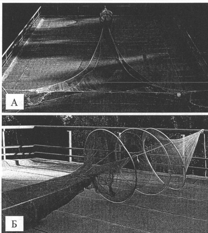
Рис. 1. Экспериментальный трал, использовавшийся при проведении съемок. А – общий вид, Б – рыбоуловитель, установленный на кутовой части трала.
